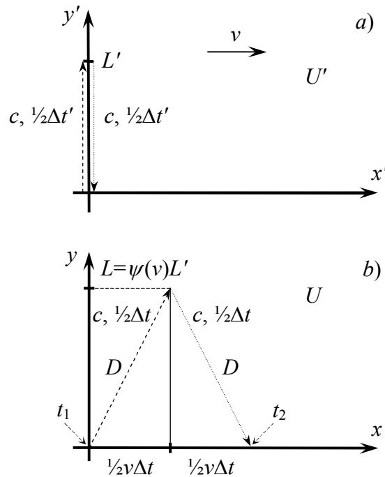
Рис. 2. Путь, проходимый светом, видимый из двух систем отсчета. a) inercjalny układ odniesienia U' , b) uniwersalny układ odniesienia U .
