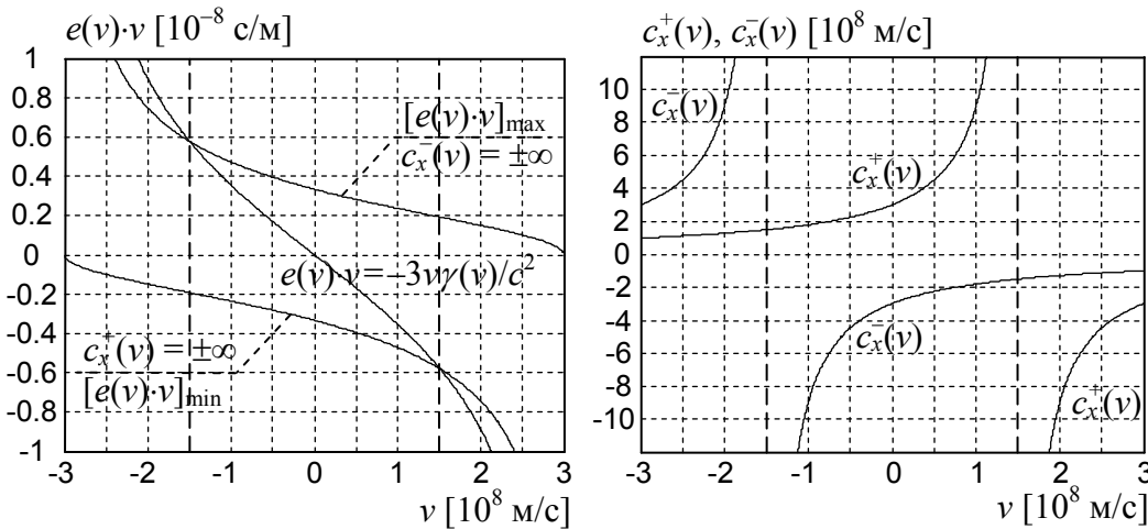
Рис. 5. Однонаправленная скорость света в вакууме как функция скорости v для e(v) \cdot v = -3v\gamma(v)/c^2 .
