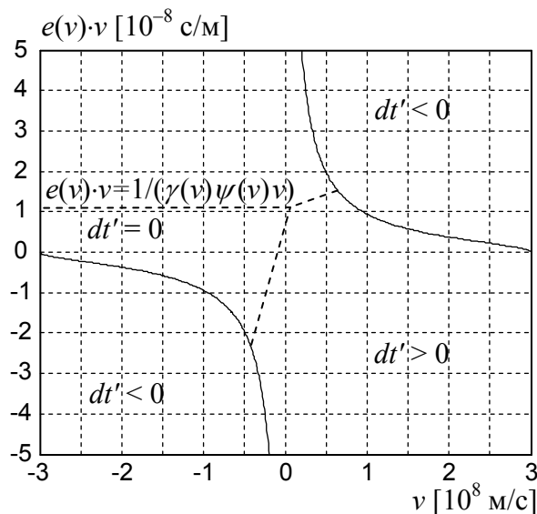
Рис. 11. Влияние значения параметра e(v) на измерение времени в движущейся инерциальной системе наблюдателем из универсальной системы отсчета ( dt > 0 ).
