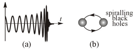
Fig. 0-24. LIGO wave.
