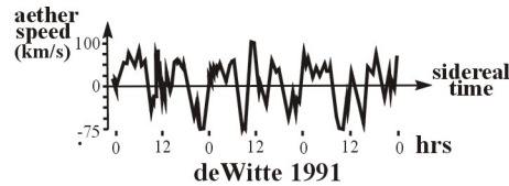
Fig. 0-21. Aether gustiness (2).
