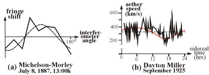
Fig. 0-20. Aether gustiness (1).
