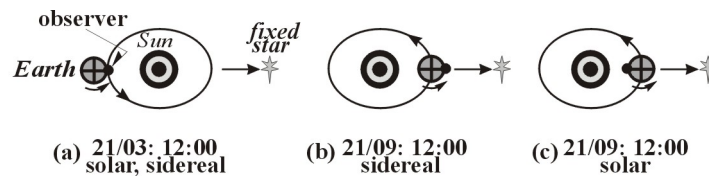
Fig. 29. Solar, sidereal times.
