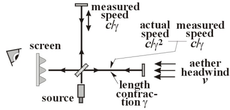
Fig. 26. Michelson-Morley (2).
