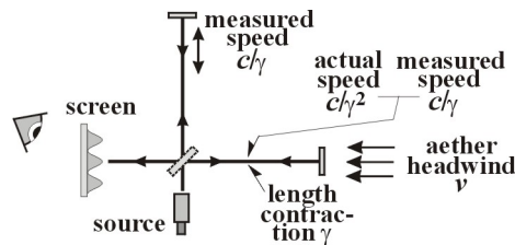
Fig. 13. Michelson-Morley (2).
