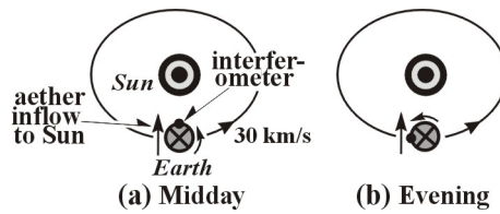
Fig. 0-22. Michelson-Morley (3).
