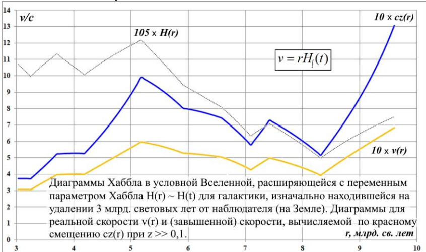
Рис.14.2. Диаграммы Хаббла для v(r) и cz(r) во Вселенной с параметром Хаббла H(r)
