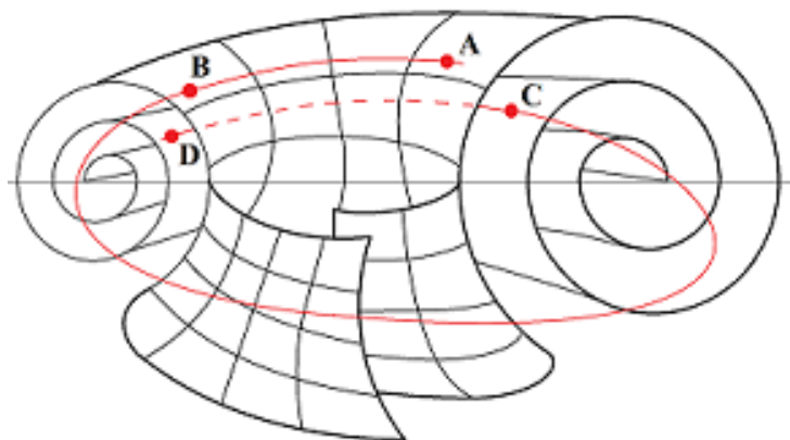
Рис.7. Тороподобная поверхность «Двойная улитка». Движение по поверхности от точки А через В и D к С происходит по спиральной геодезической
